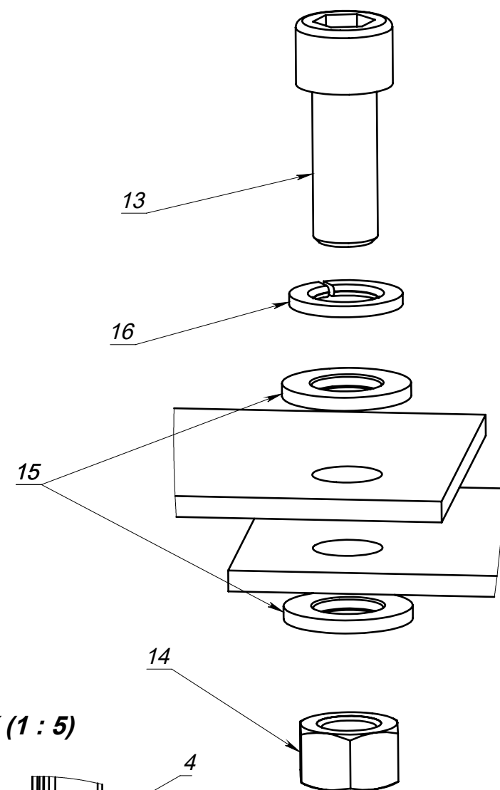
Varžtinio sujungimo surinkimas
