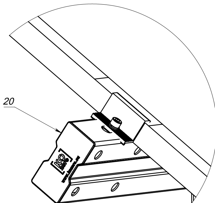
Kamščių tvirtinimas (1 : 3)
