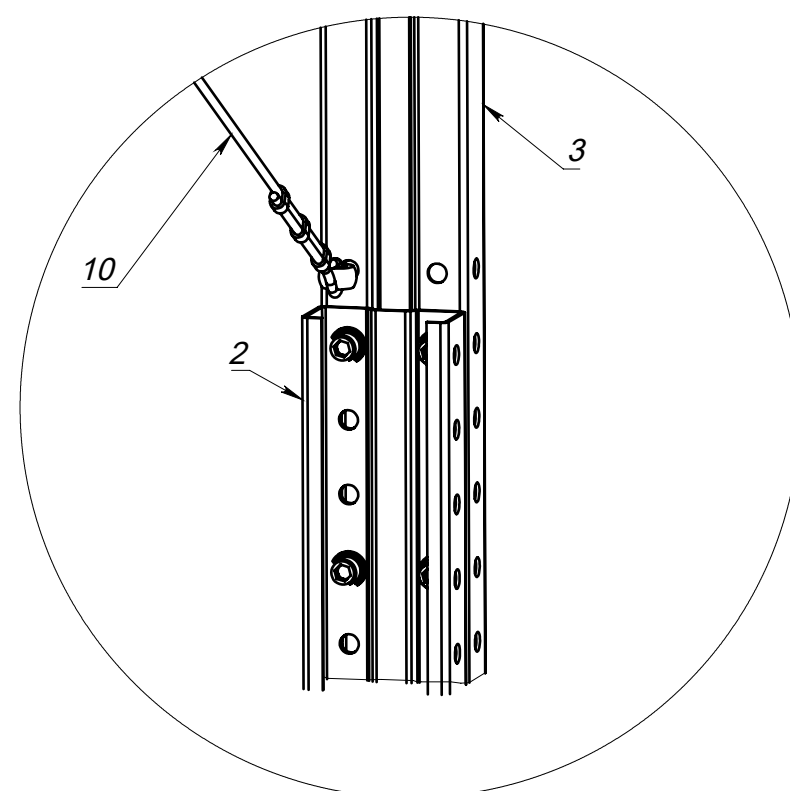
IX (1 : 5)
