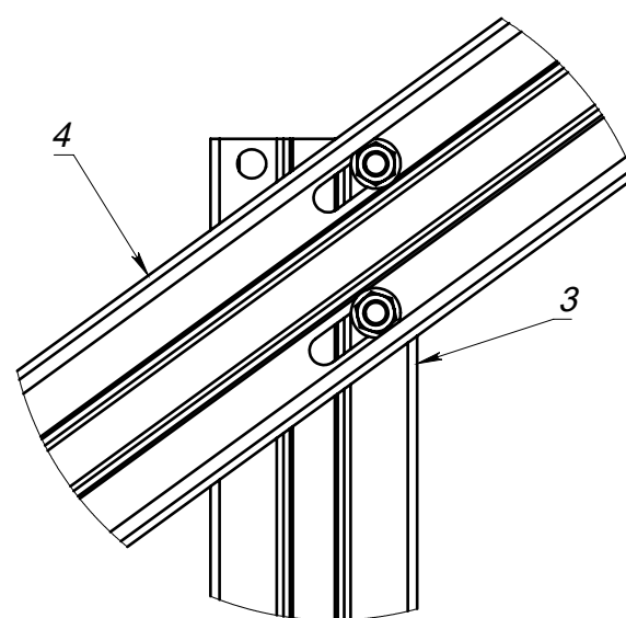
VII (1 : 4)
