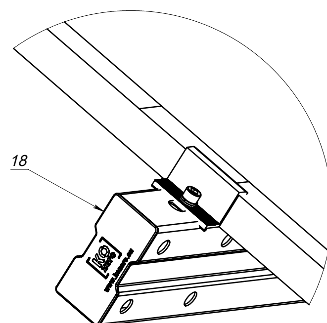
IX (1 : 5)
