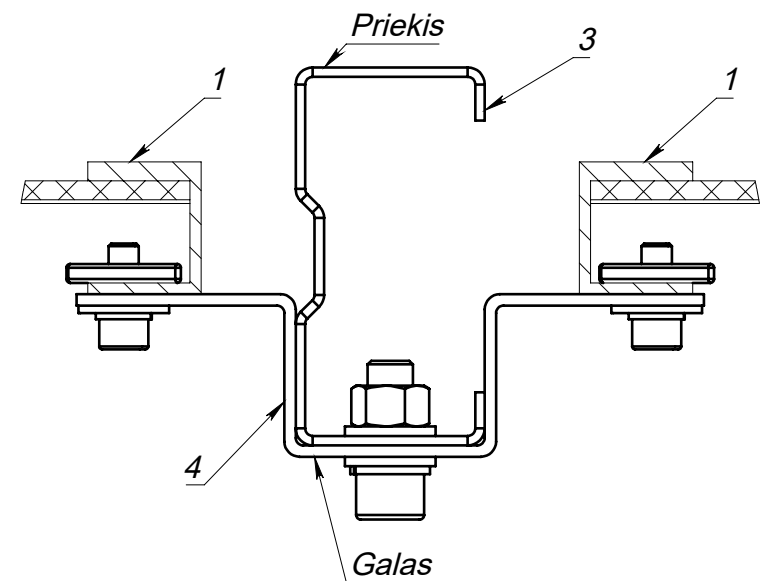
III (1 : 2) iš viršaus
